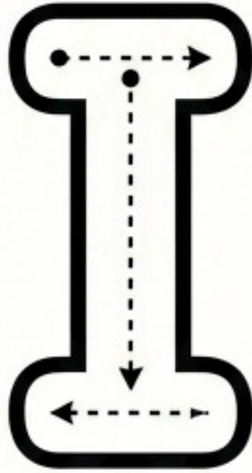
Uppercase I
